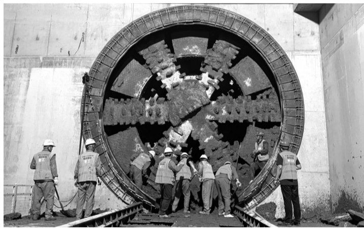
施工现场 无锡地铁供图
