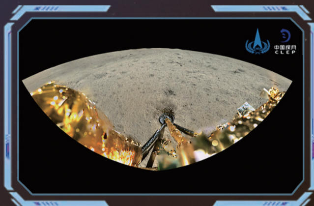
嫦娥六号着陆器全景相机拍摄的全景镶嵌图
