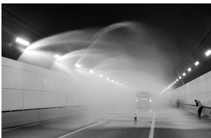
隧道消防喷淋系统测试 通讯员供图
