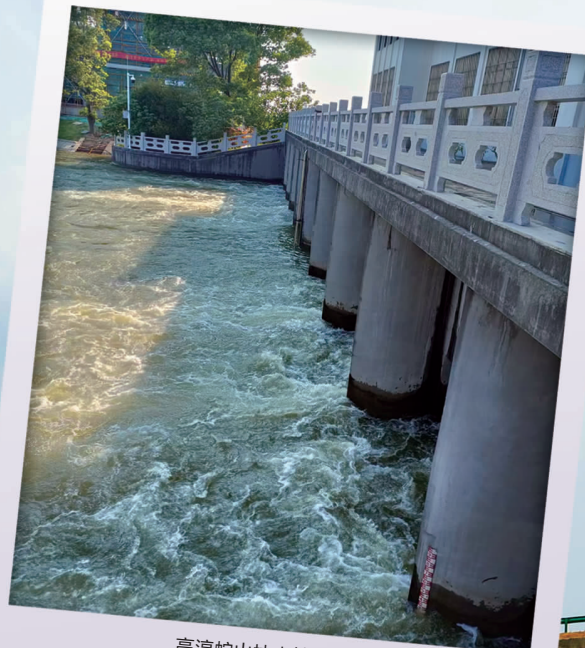
高淳蛇山抽水站出水 南京市水务局供图
