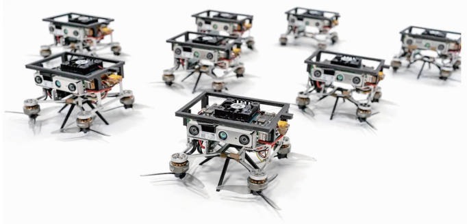
微型空中机器人 浙江大学供图
