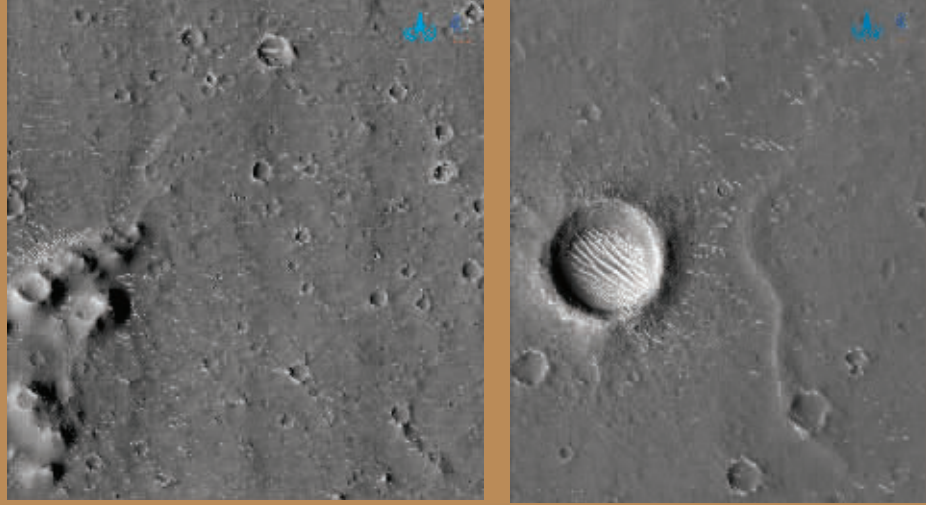
3月4日,国家航天局发布3幅由我国首次火星探测任务“天问一号”探测器拍摄的高清火星影像图,包括2幅全色图像和1幅彩色图像 新华社发
