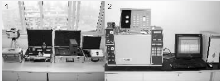
1.全套检测仪器 从左至右依次为：双气路大气采样仪、TVOC检测仪、甲醛检测仪、氢分析仪 2.气相色谱仪 主要作用：后期采样数据分析
