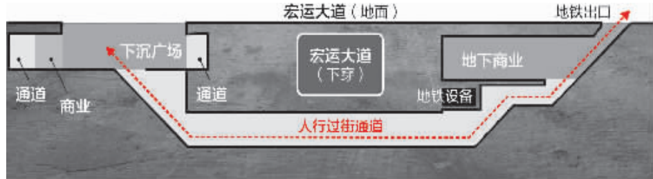
宏运大道下穿通道剖面图 制图 李荣荣
