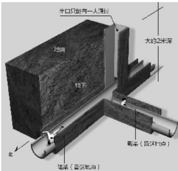
事发下水道切面示意图 制图 李荣荣
