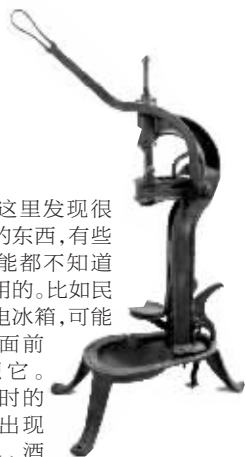
民国时的压力打盖封装机
