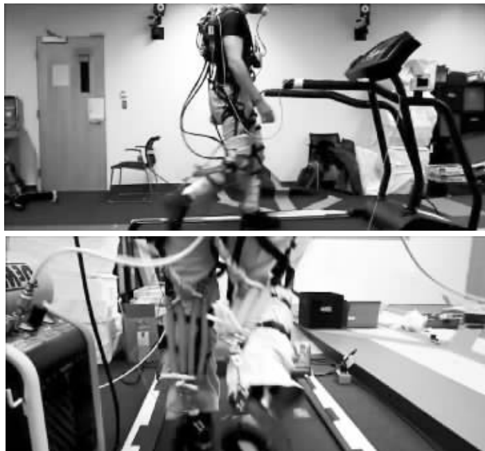
实验对象穿着机械服在跑步机上进行测试
