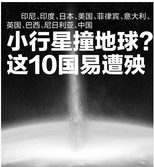
行星撞入地球(模拟图)
