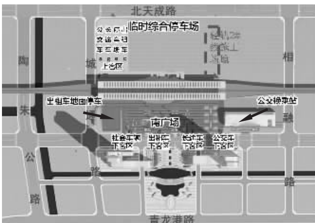
苏州北站临时旅客流线图
