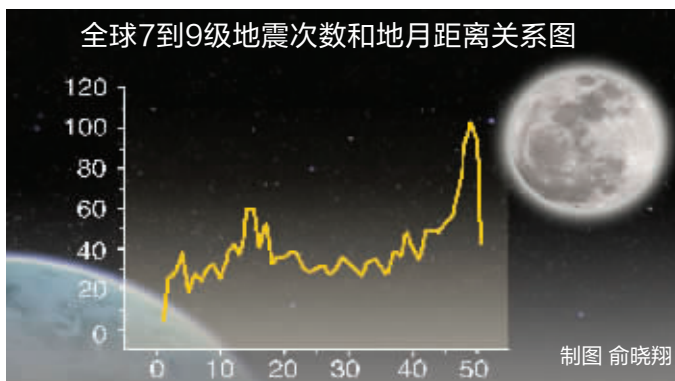
纵轴是1900年至2011年3月11日间全球7级以上地震次数,横轴是地月距离区间(将地月距离从356000公里到407000公里划分为51等份)
