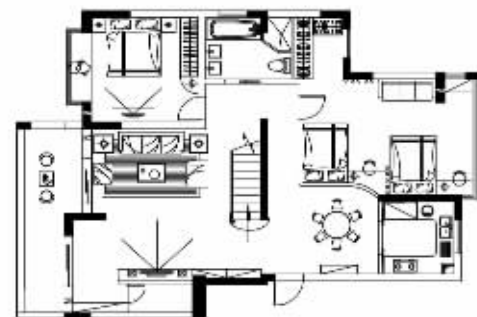
一层平面图
