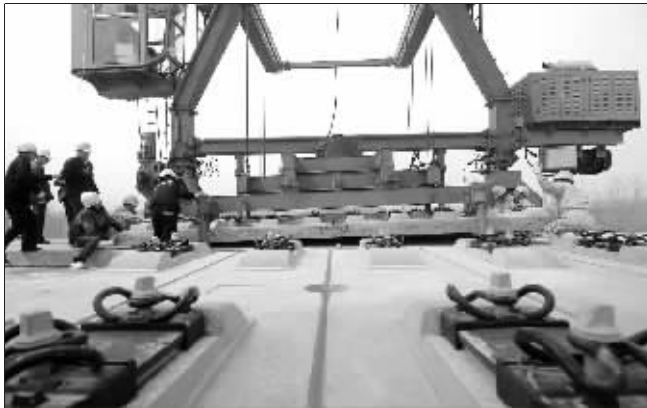
3月17日,中铁十二局京沪高铁四标段开始轨道板铺设准备作业 新华社记者 刘军喜 摄
