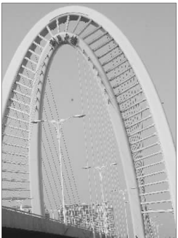
宜兴荆邑大桥近日建成通车。该大桥长544.5米,桥面为双向8车道,最宽达58.5米,是目前国内桥面最宽的封闭式钢箱梁桥,充满时代气息,十分壮观。 闵学平 陈超
