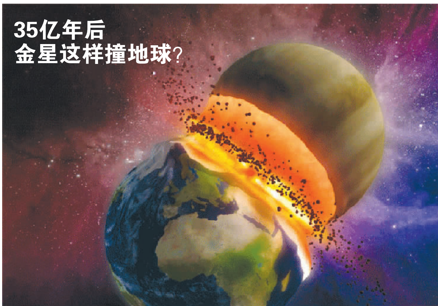
英国《自然》期刊6月10日发表一项最新研究称,一种叫做“轨道混沌”的力量可能致使地球与金星、火星等相撞,从而引发太阳系混乱。但这种混乱出现几率极低,且至少是在35亿年后。是否出现轨道混沌的关键取决于太阳系内距离太阳最近的星球——水星。在先前研究中,天文学家能够准确估算未来数百年、数千年太阳系发展状况。但像这样推算更长时间太阳系发展情况的实验尚属首次。这是《自然》出版集团提供的地球与金星相撞的模拟图。新华社/法新
