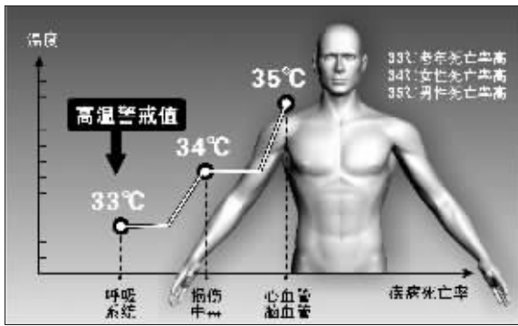
温度与死亡率的关系 李荣荣 制图
