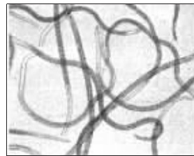
松材线虫
