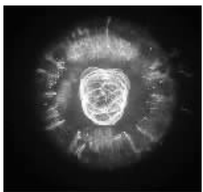
第三美景:爱斯基摩星云
